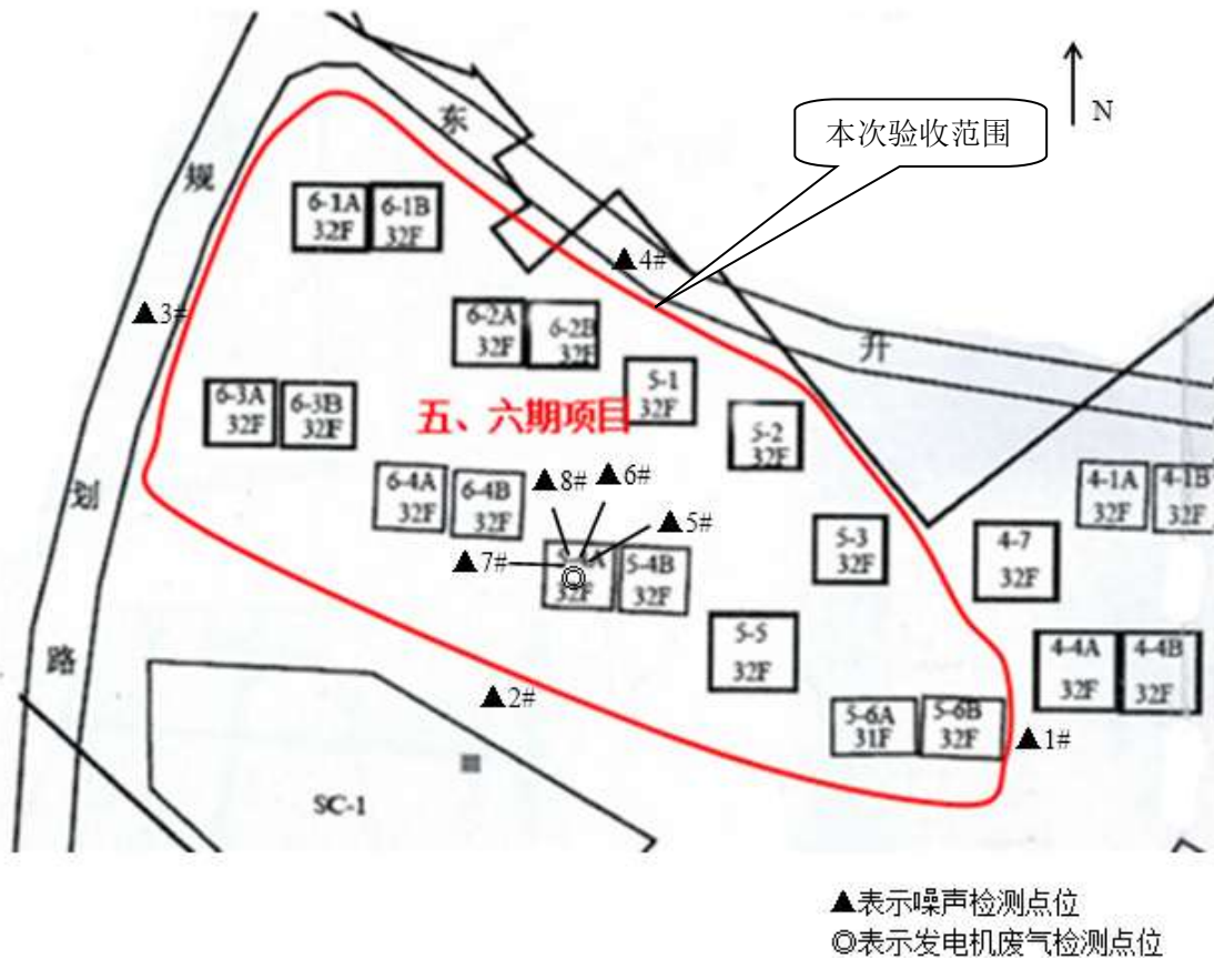
图 8.2-1 建设项目噪声及废气监测点位示意图
